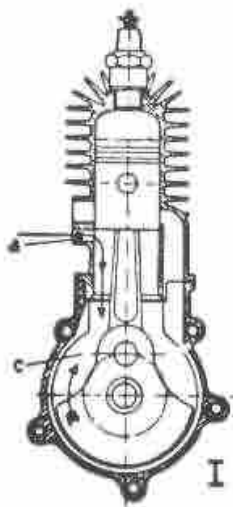
Bild 2.2 Einlassen
