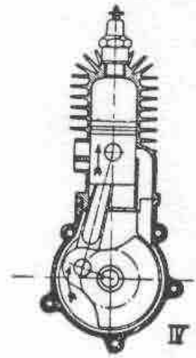
Bild 2.5 Verdichtung
