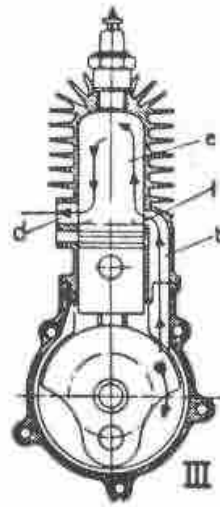
Bild 2.4 Spülung
